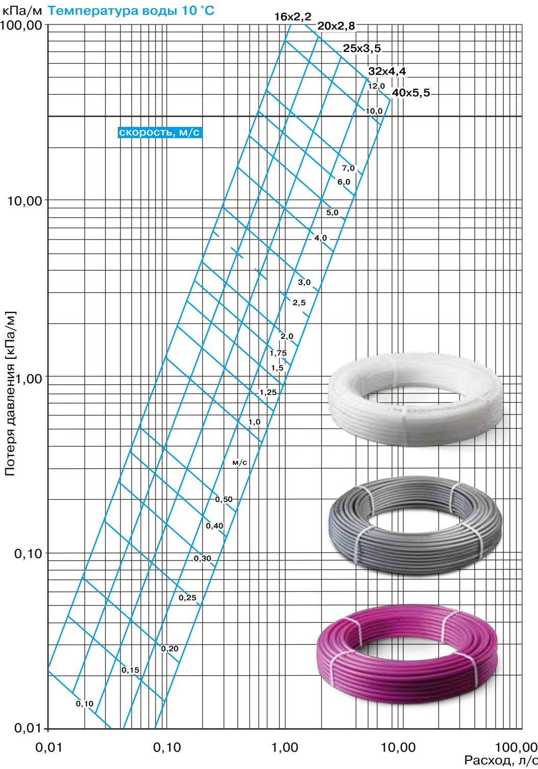
1. График линейных потерь давления в трубах PRO AQUA PE-Ха (серебристая) SDR 7.4 и PE-RT SDR 7.4 (белая)
