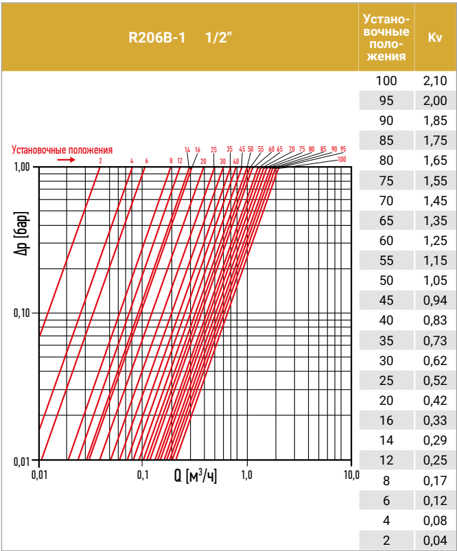
Диаграмма зависимости потерь давления от расхода по линии С-Д с отводом Ду 15 при установке ремонтной вставки
