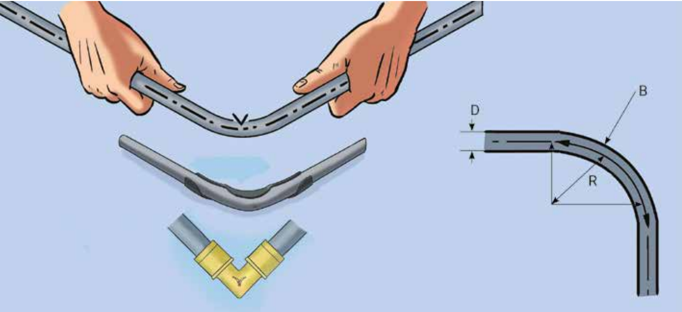
Минимальный радиус изгиба при изгибании вручную ( R = 8 \times D )
