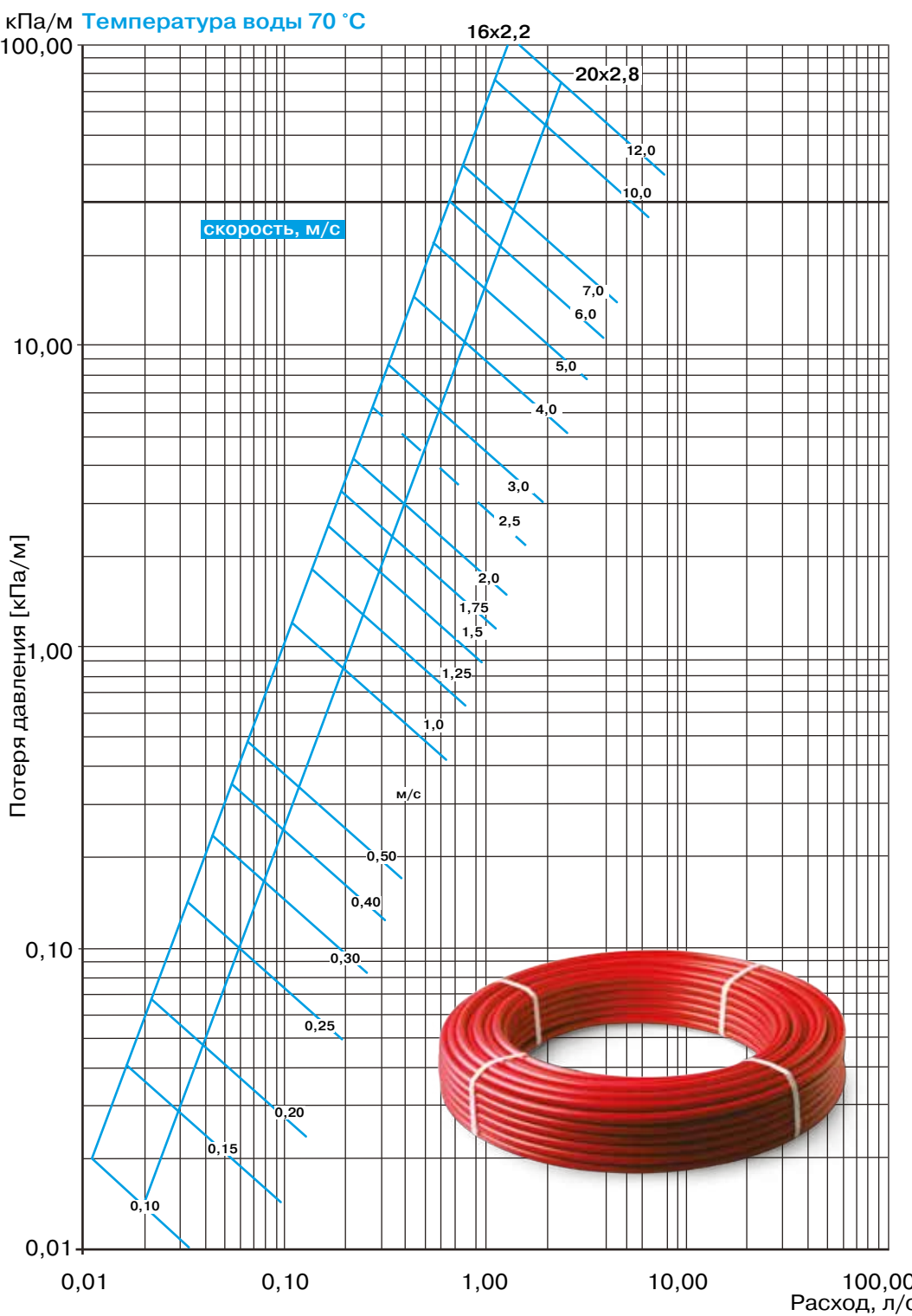
2. График линейных потерь давления в трубах PRO AQUA PE-Ха (красная), S3.5 / S4.5
